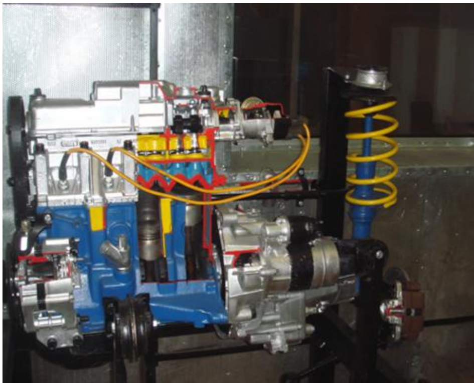
Учебные экспонаты: Разрез двигателя легкового автомобиля
