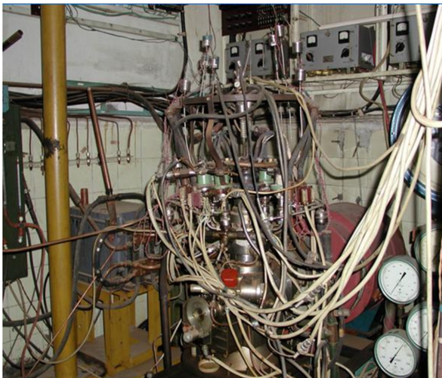
Лабораторная установка: Стенд с двигателем Стирлинга
